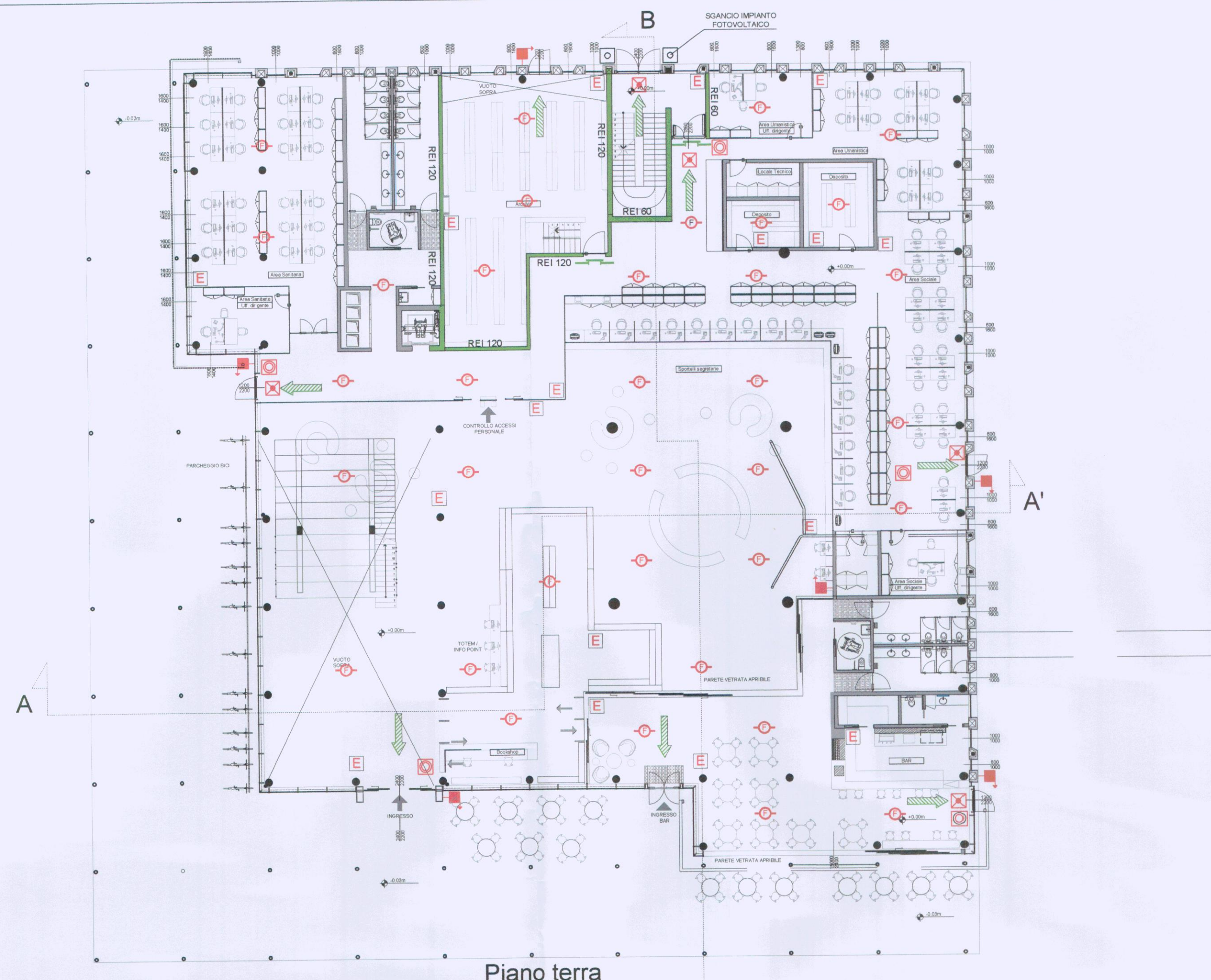
Piano terra scala 1:200
